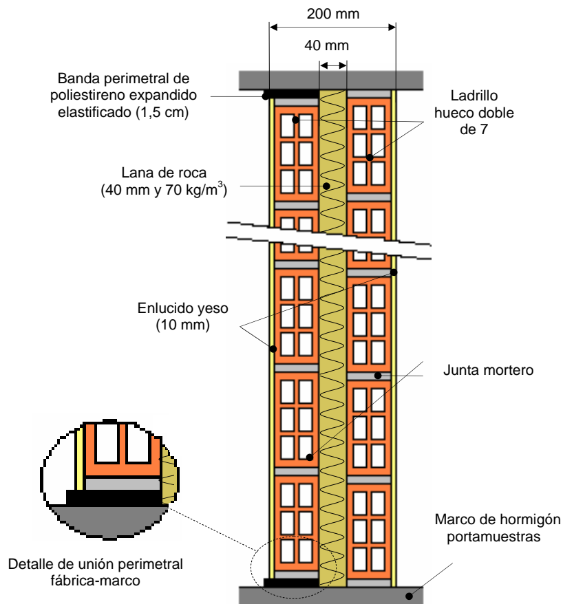
Figura 1: Esquema de la muestra ensayada (B0103-03-M116)
