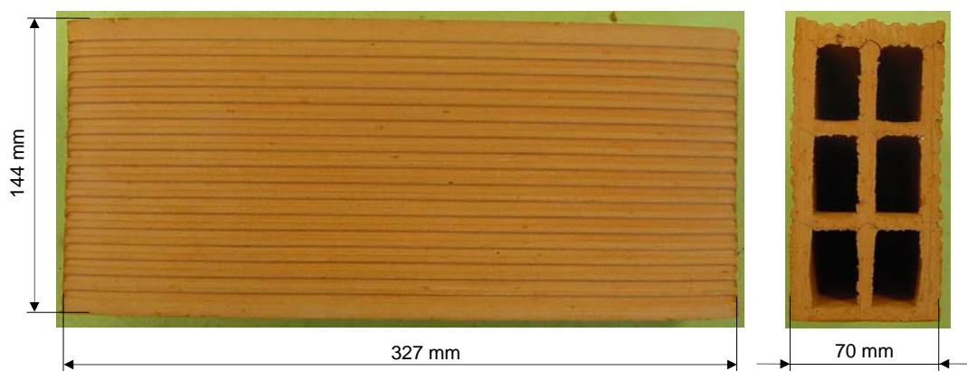
Figura 2: Dimensiones medidas del ladrillo hueco doble de 7
