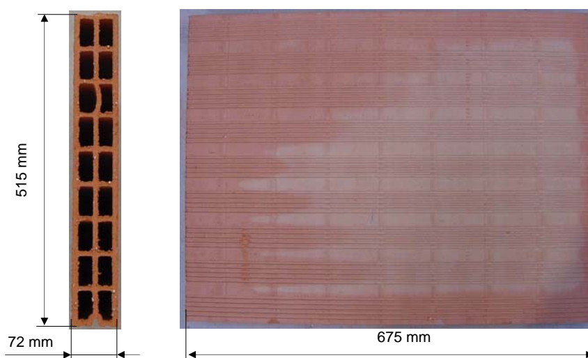
Figura 2: Dimensiones medidas del ladrillo gran formato de 7
