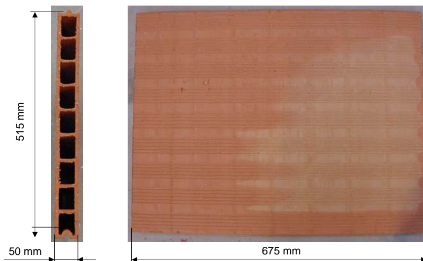
Figura 3: Dimensiones medidas del ladrillo gran formato de 5
