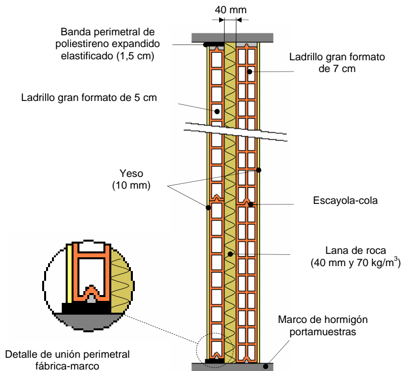
Figura 1: Esquema de la muestra ensayada (B0103-03-M122)
