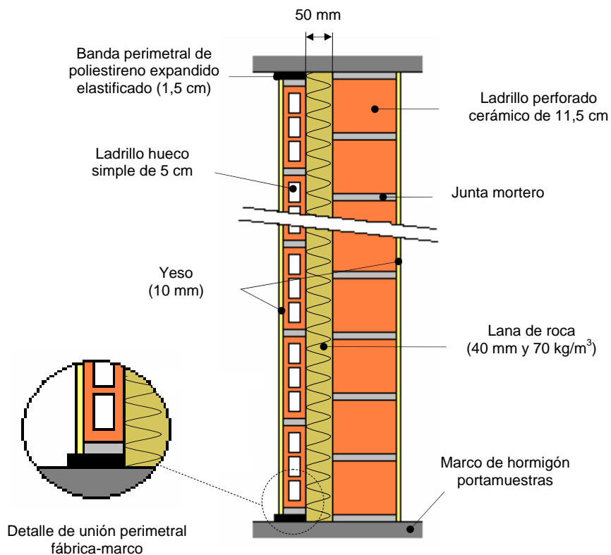
Figura 1: Esquema de la muestra ensayada (B0103-03-M114)
