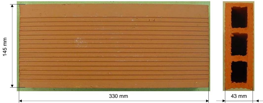
Figura 3: Dimensiones medidas del ladrillo hueco simple de 5
