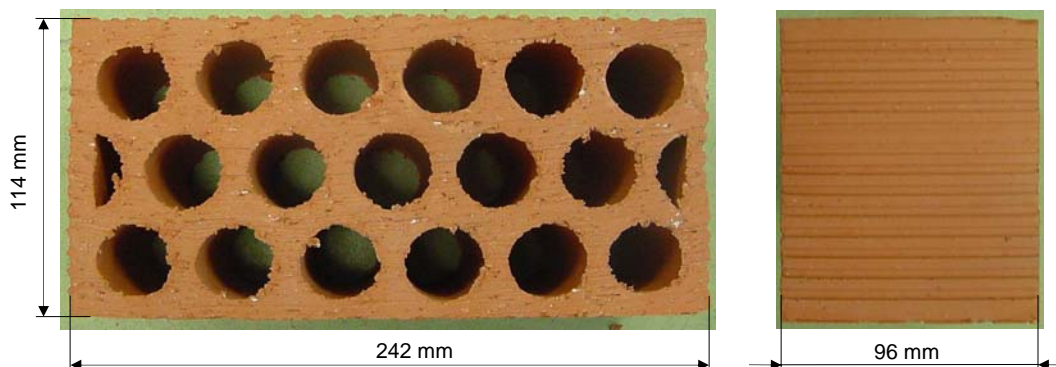
Figura 2: Dimensiones medidas del ladrillo perforado cerámico de 11,5
