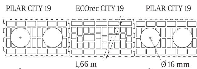
PIEZA ESPECIAL para RETRANQUEO - ARRANQUE PILAR CITY 19
