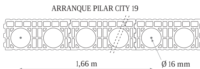
PIEZA ESPECIAL para RETRANQUEO - ARRANQUE PILAR CITY 19
