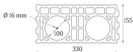
PIEZA ESPECIAL para RETRANQUEO - ARRANQUE PILAR CITY 19
